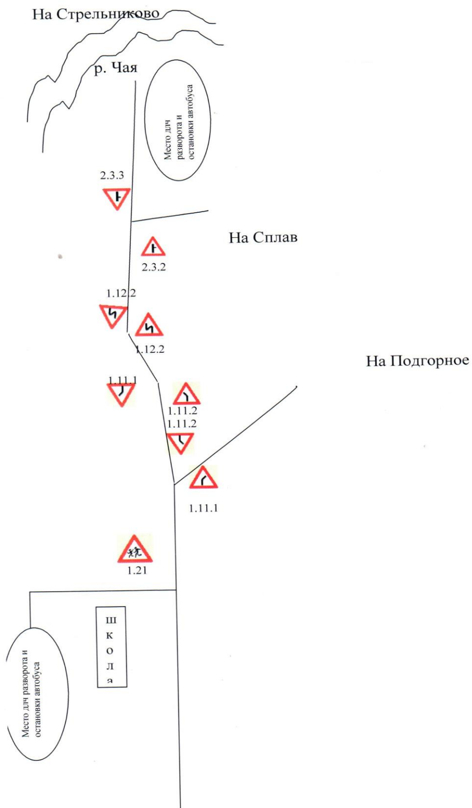
Схема маршрута перевозки Варгатер – Стрельниково - Варгатёр
